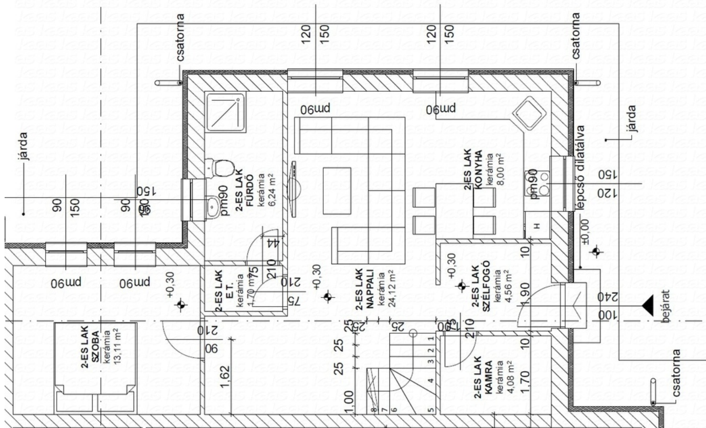
Földszint alaprajz
