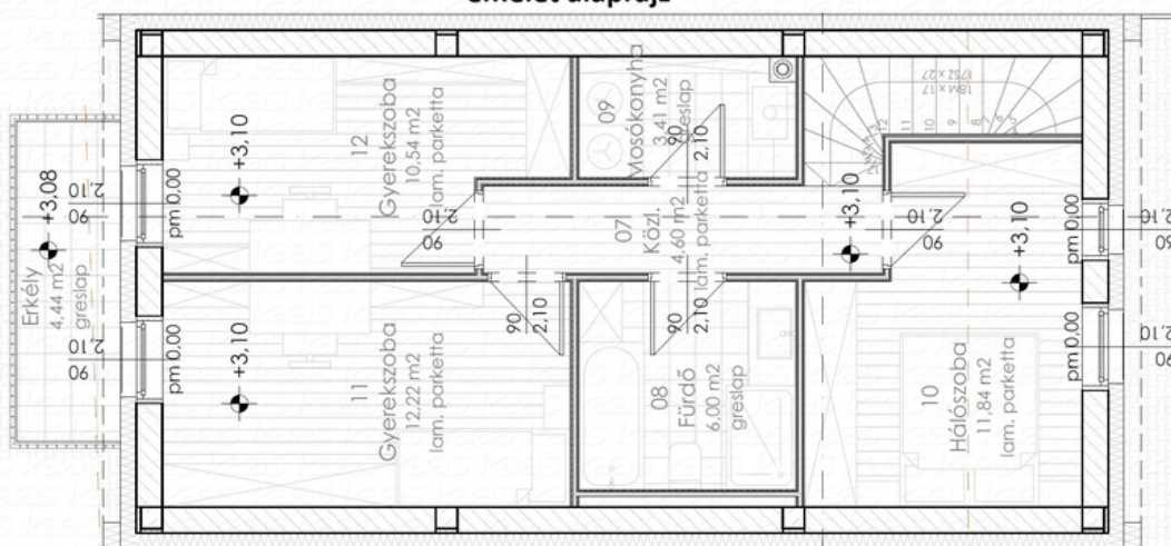
emelet alaprajz
